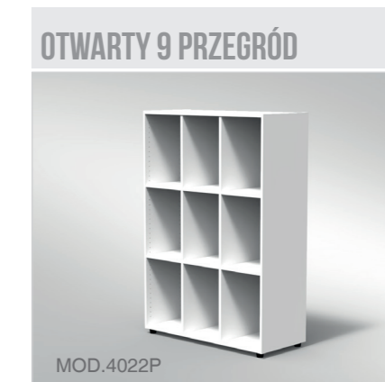
■ REGAŁ OTWARTY 9 PRZEGRÓD 6 PÓLEK ■ WYMIARY: 104x44x150h.
