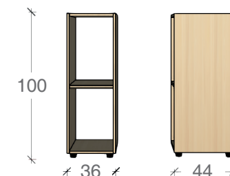
DIMENSIONI esterne: 36x44x100h. cm
