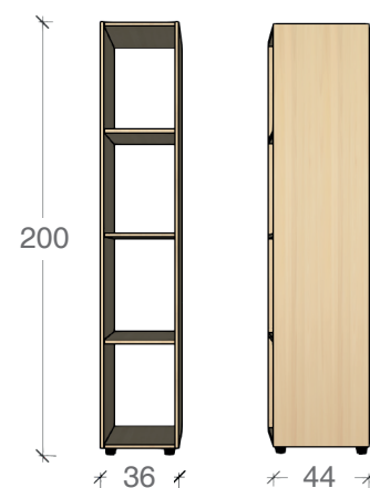
DIMENSIONI esterne: 36x44x200h. cm
